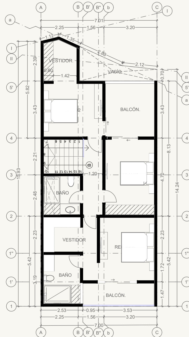
ARQ. PLANTA ALTA. 1:50
